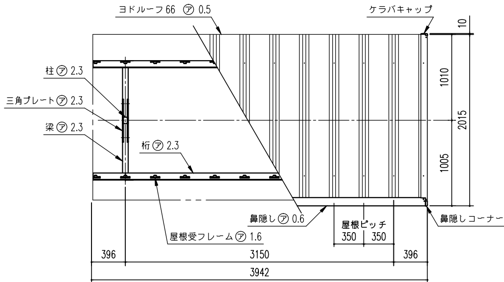
小屋伏図 (S=1/30)
