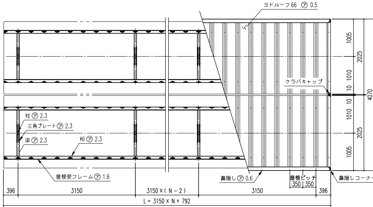
小屋伏図 (S=1/40)
