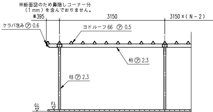
正面断面図 (S=1/40) (N: スパン数)
