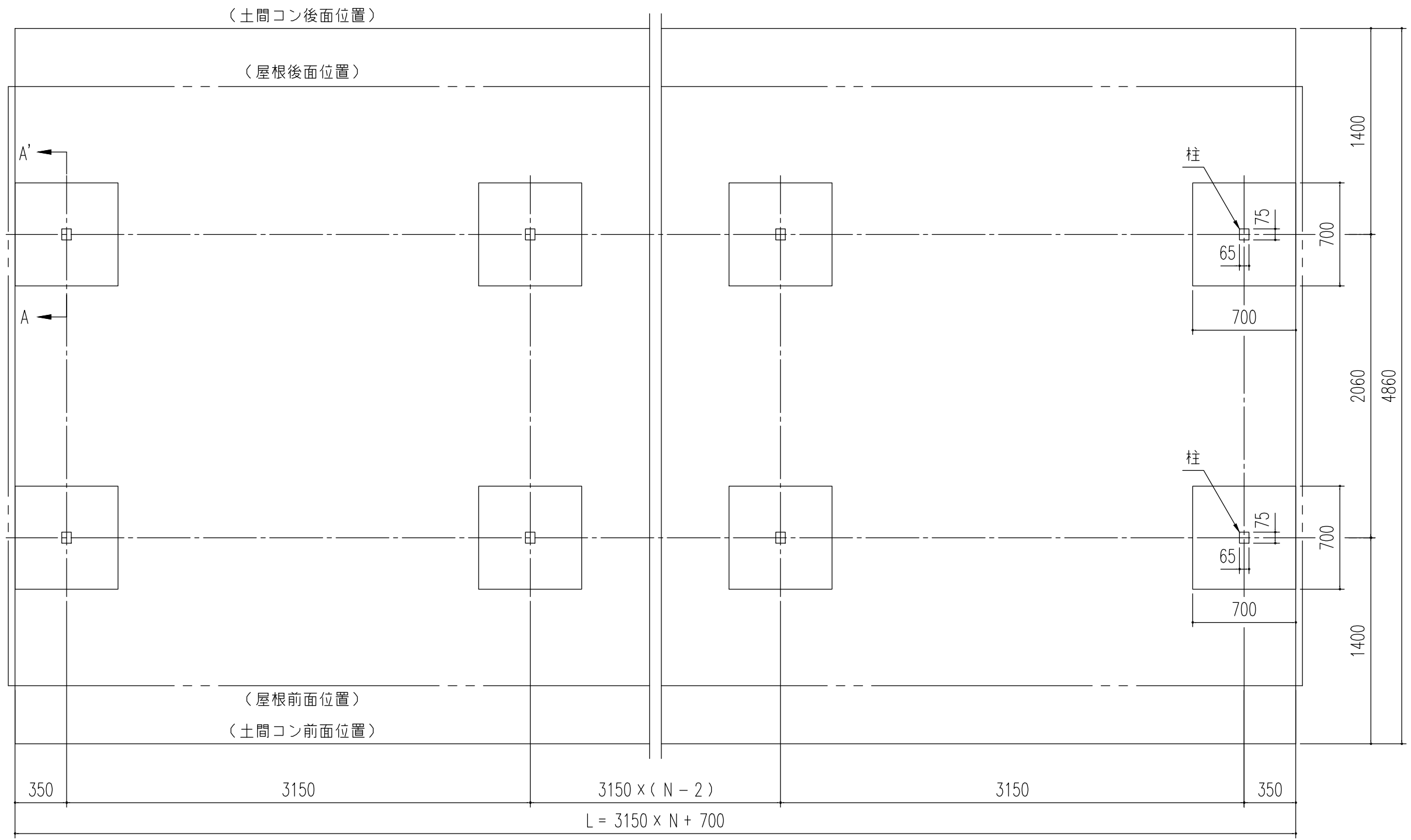
基礎伏図 (S=1/30) (N: スパン数)
