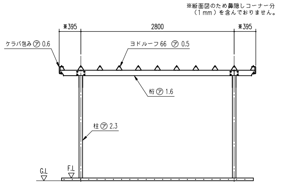
正面断面図 (S=1/30)
