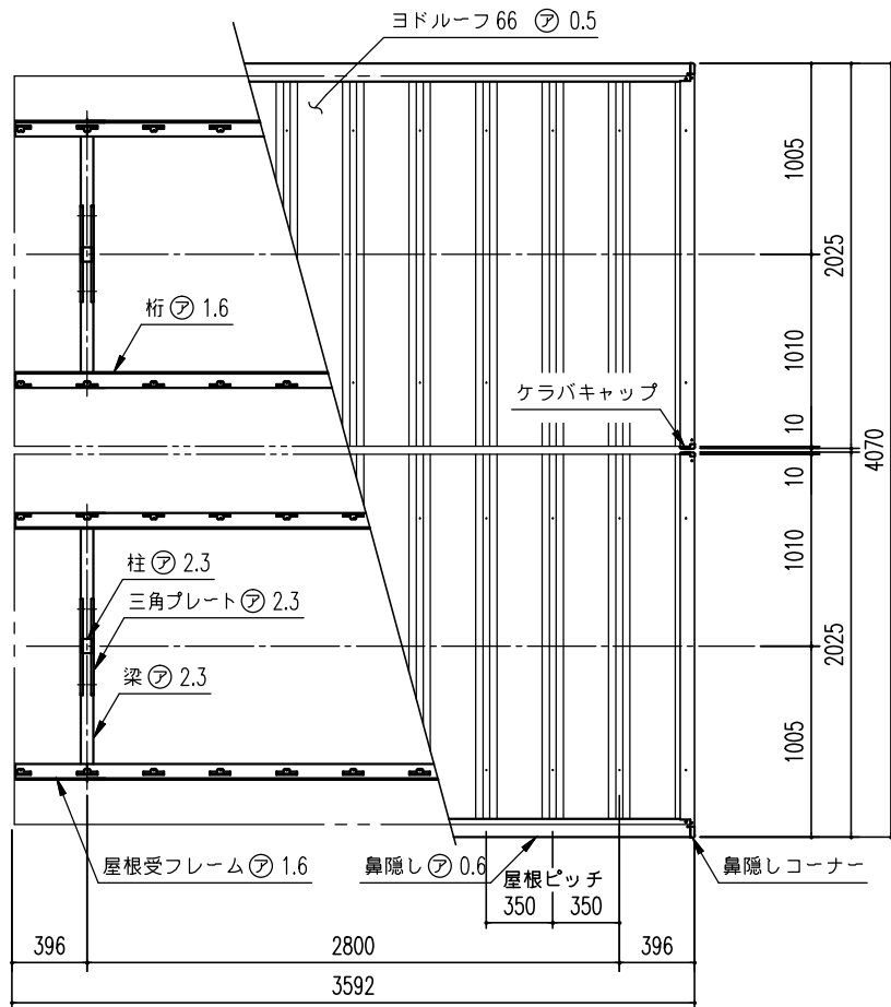
小屋伏図 (S=1/30)
