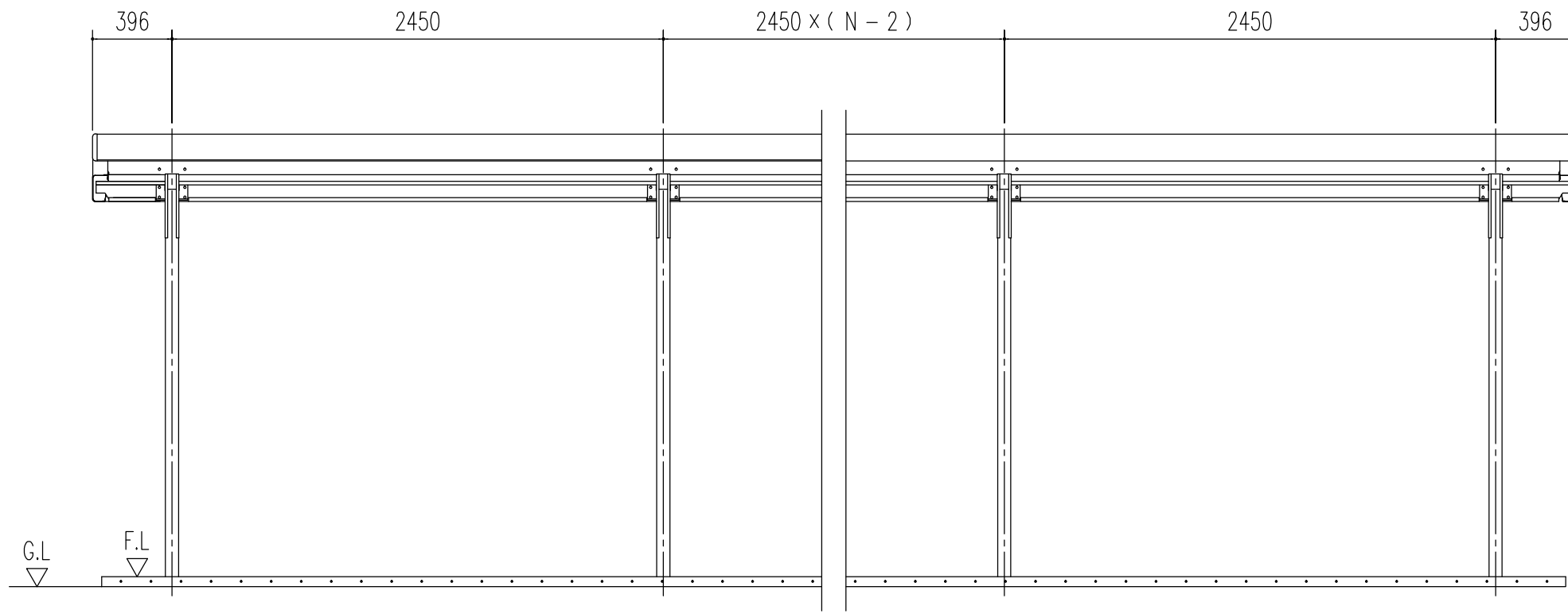
正面立面図 (S=1/30) (N: スパン数)
