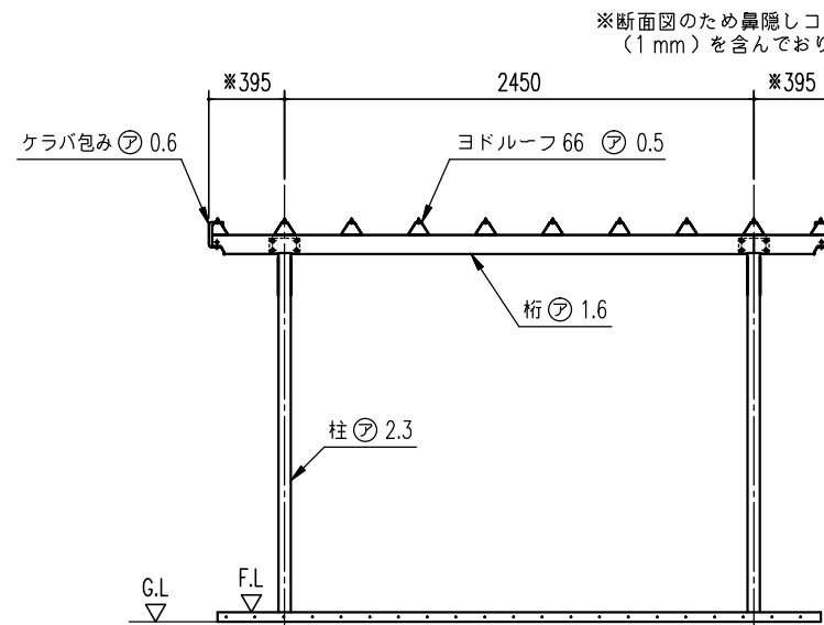
正面断面図 (S=1/30)
