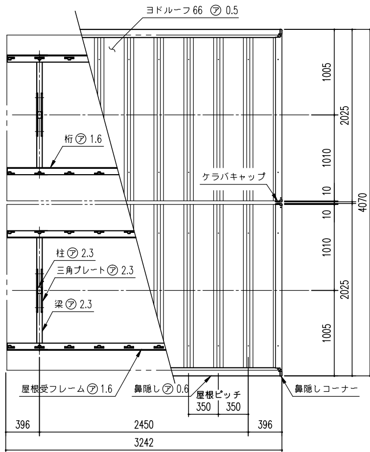
小屋伏図 (S=1/30)
