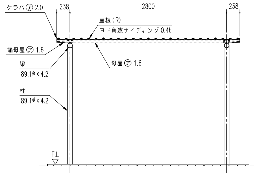
正面断面図 (S=1/40)
