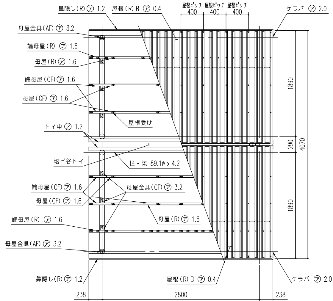
小屋伏図 (S=1/40)
