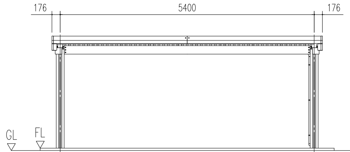
正面立面図 (S= 1/50)
