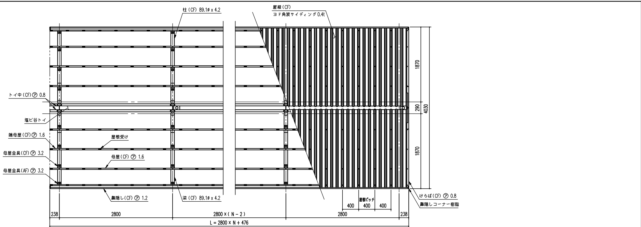
小屋伏図 (S=1/40)
