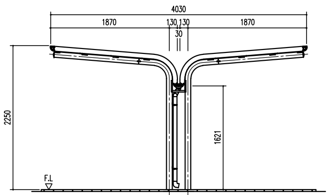
側面立面図 (S=1/40)
