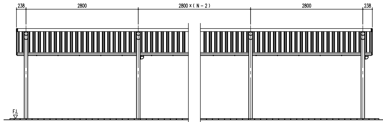
正面立面図 (S=1/40) (N : スパン数)
