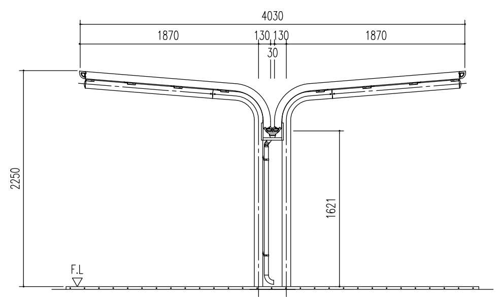
側面立面図 (S=1/40)
