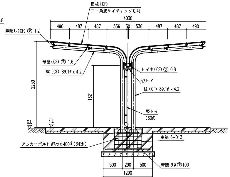
側面断面図 (S=1/40)
