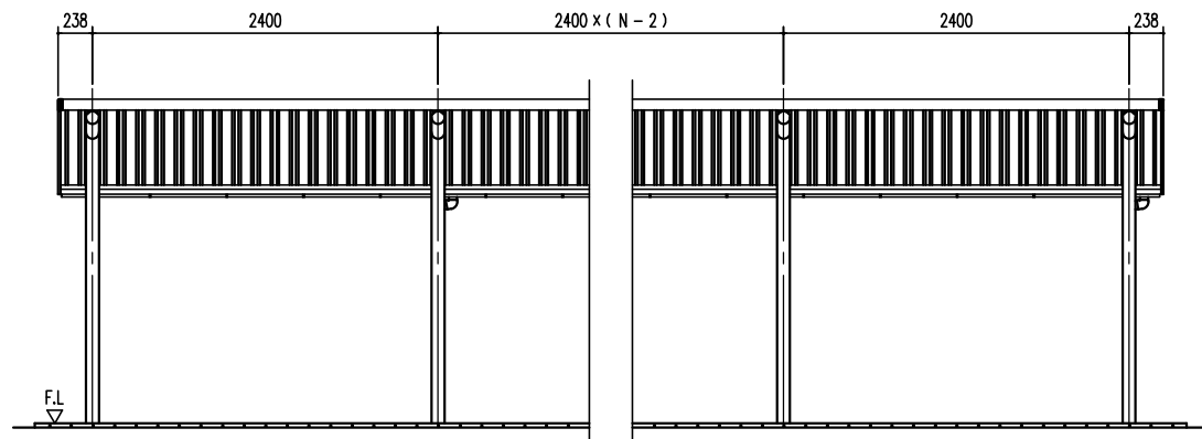
正面立面図 (S=1/40) (N: スパン数)
