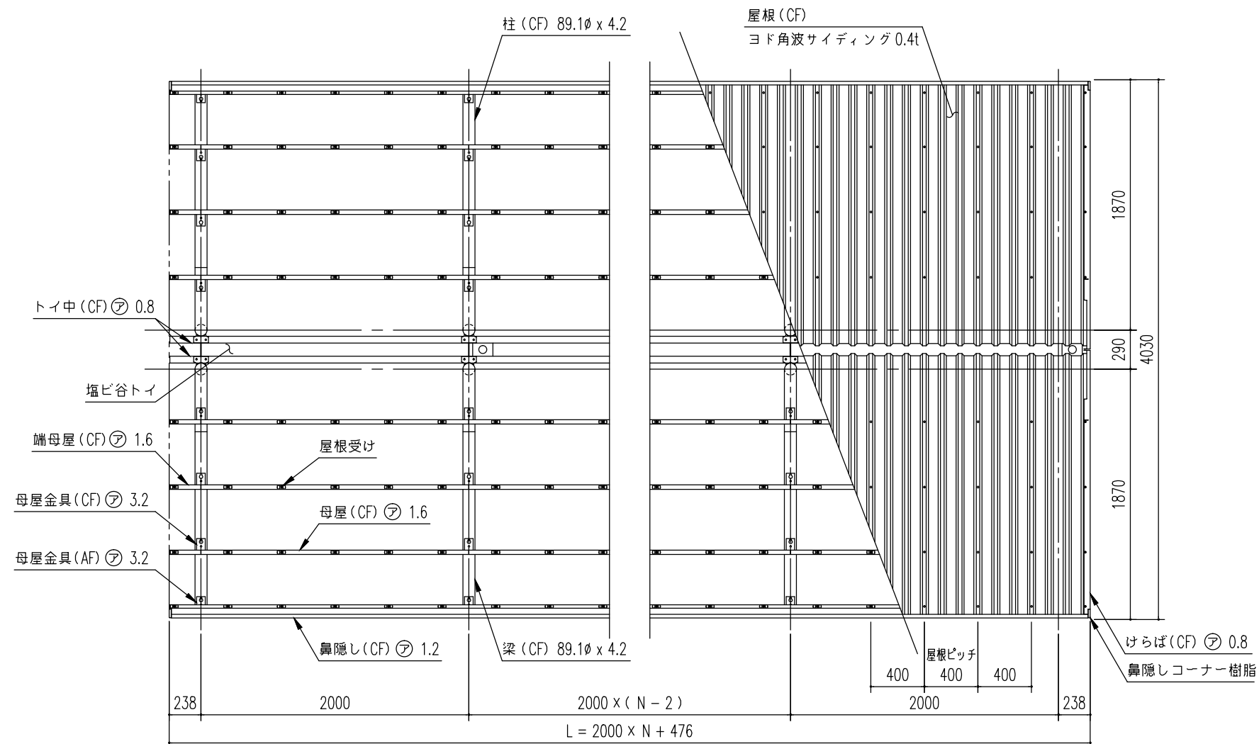
小屋伏図 (S=1/40)
