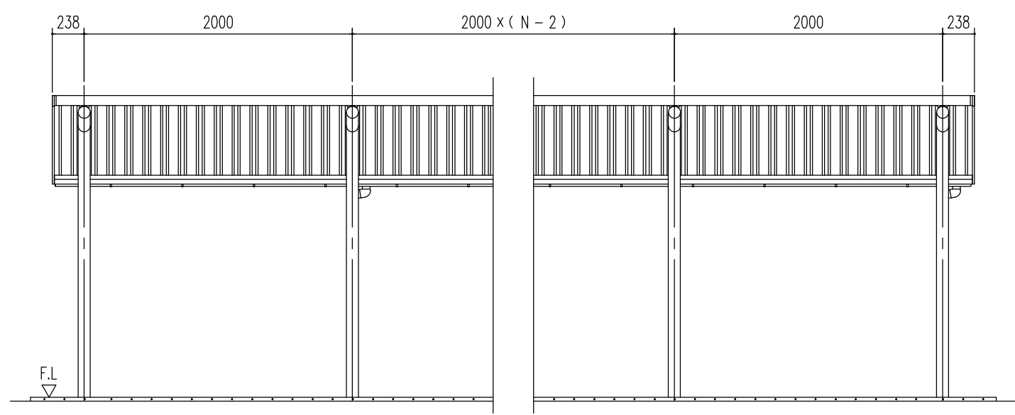
正面立面図 (S=1/40)
