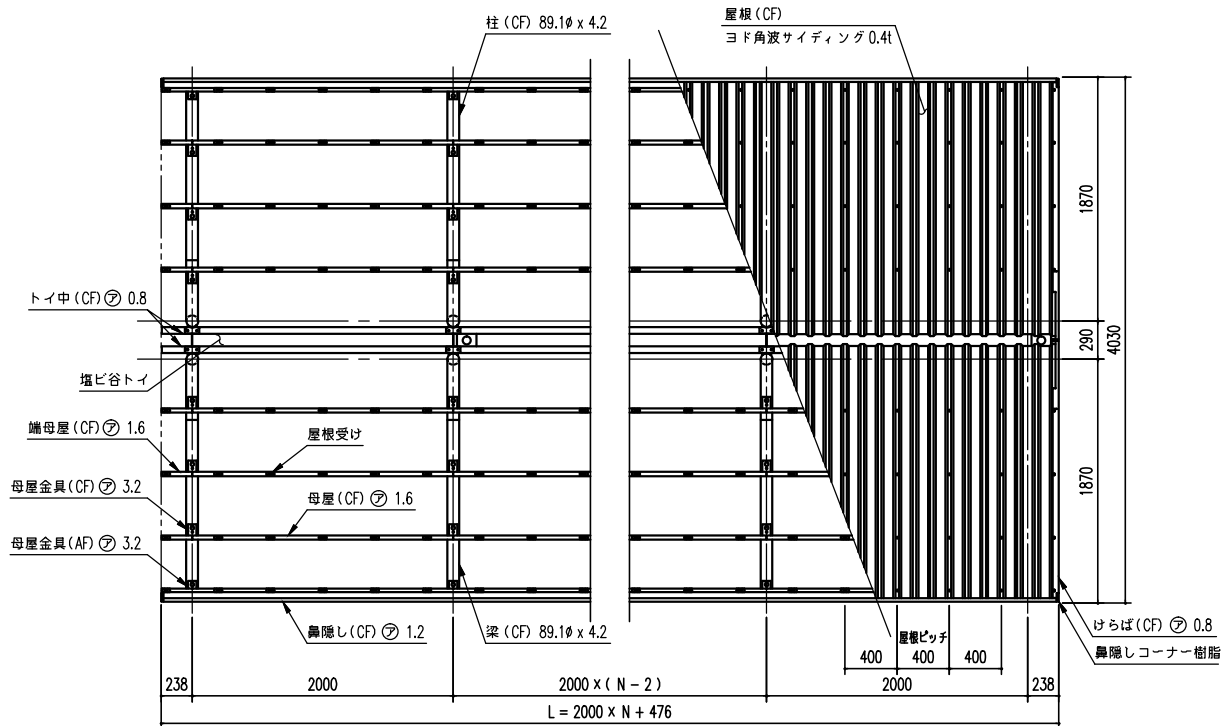
小屋伏図 (S=1/40)
