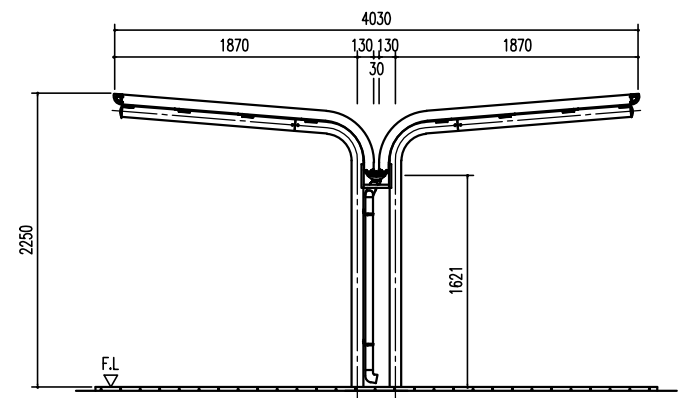
側面立面図 (S=1/40)
