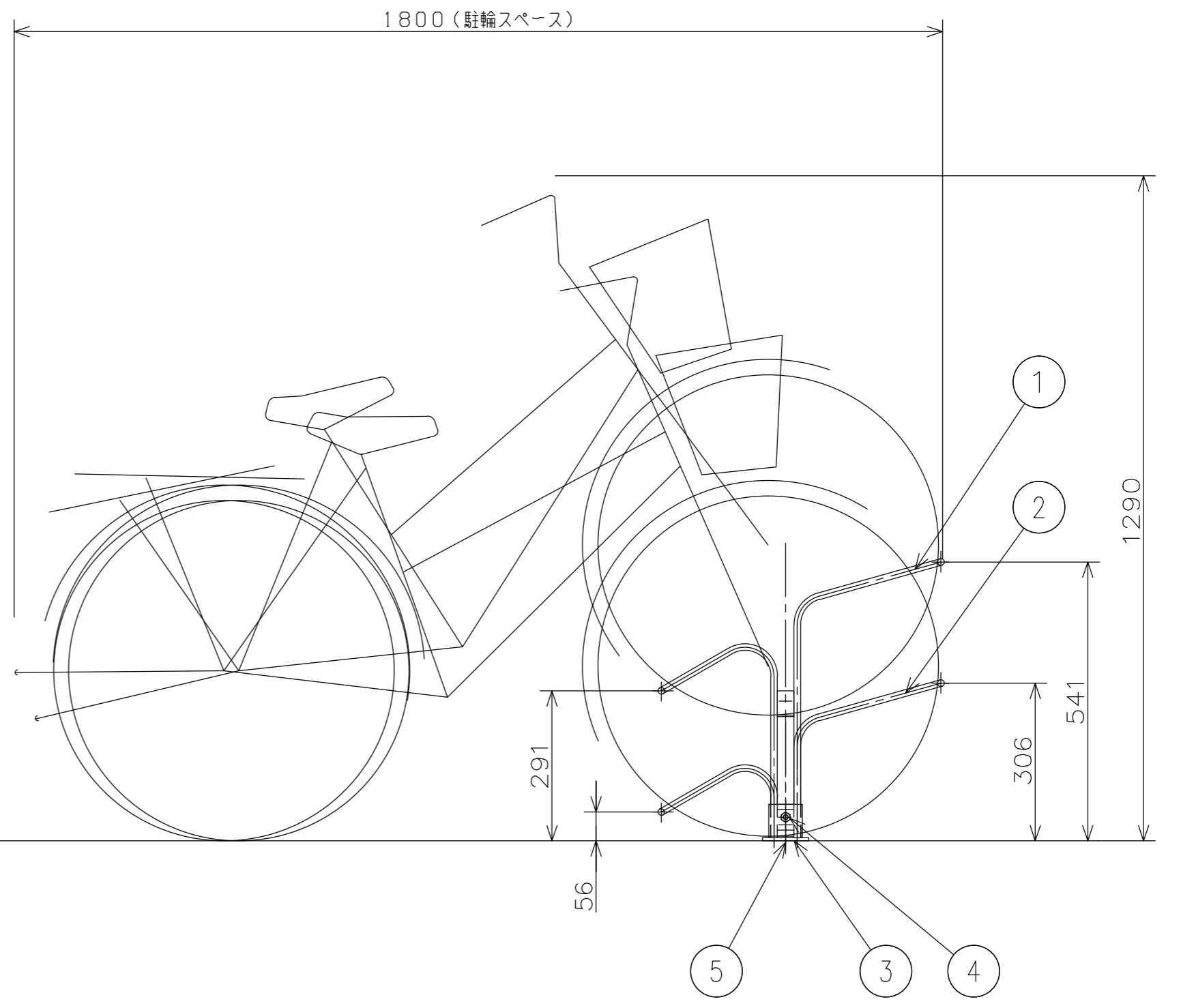
側面図 1:10
