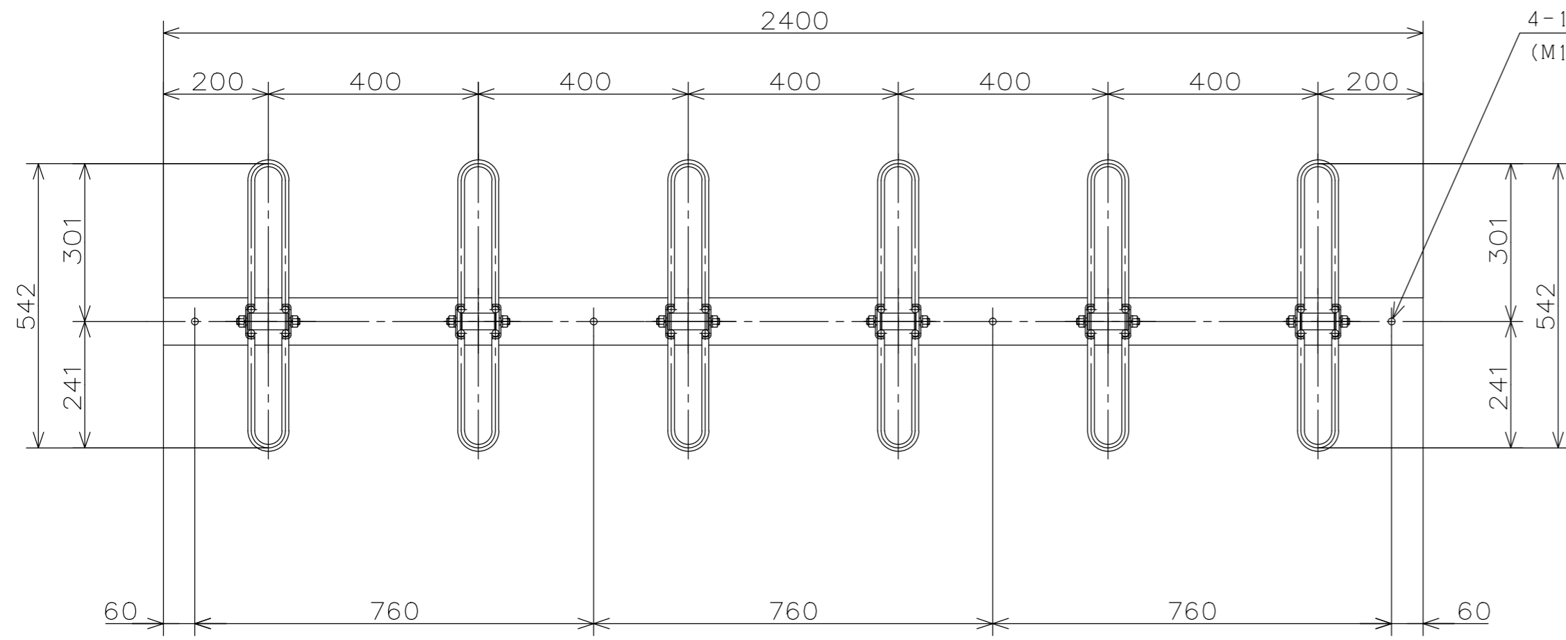
平面図 1:10
