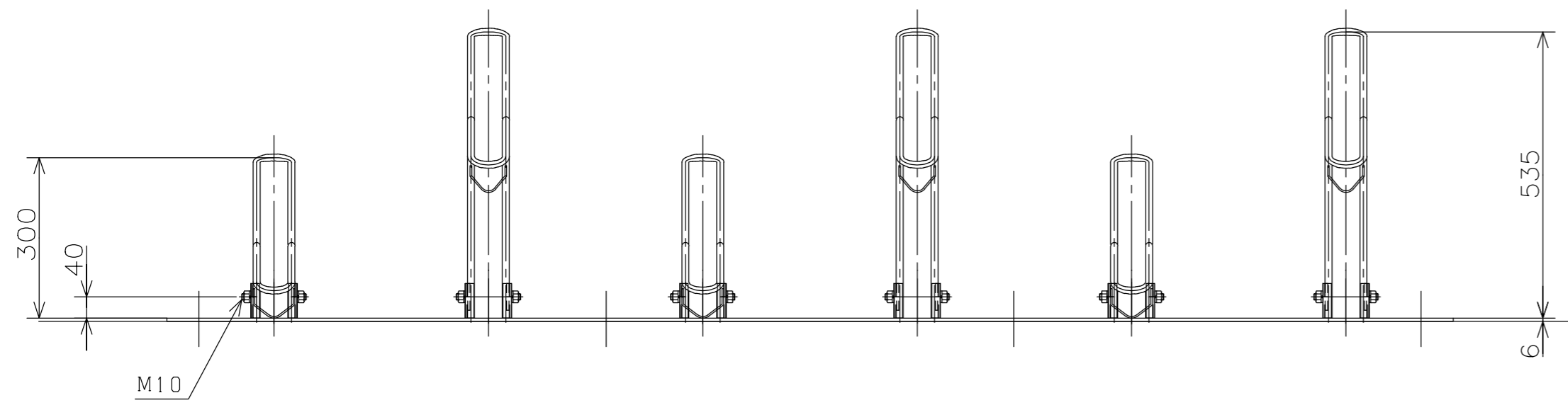
立面図 1:10
